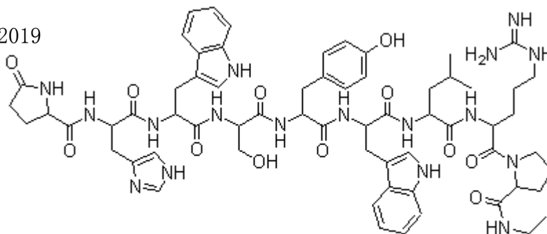
Pyr-His-Trp-Ser-Tyr-D-Trp-Leu-Arg-Pro-NHEt
